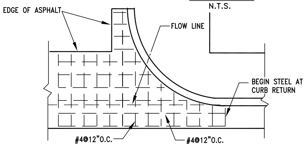
DETAIL B N.T.S.
